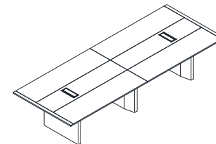
A款会议桌 PJE-MTA-3613 尺寸: 3600W*1350D*760H
